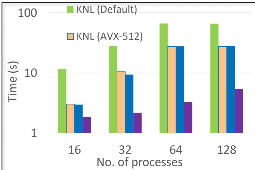
DAXPY kernel
