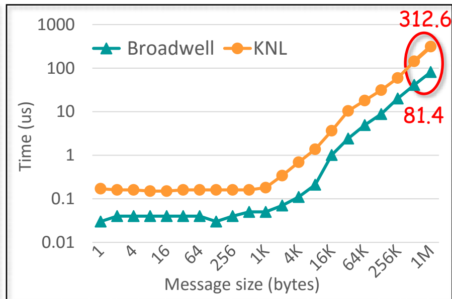
Shmem_getmem
